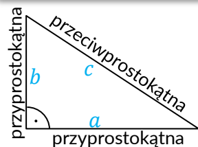
trójkąt prostokątny
