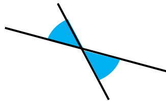
kąty wierzchołkowe
