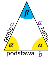
trójkąt równoramienny
