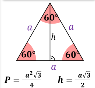
wielokąt foremny
